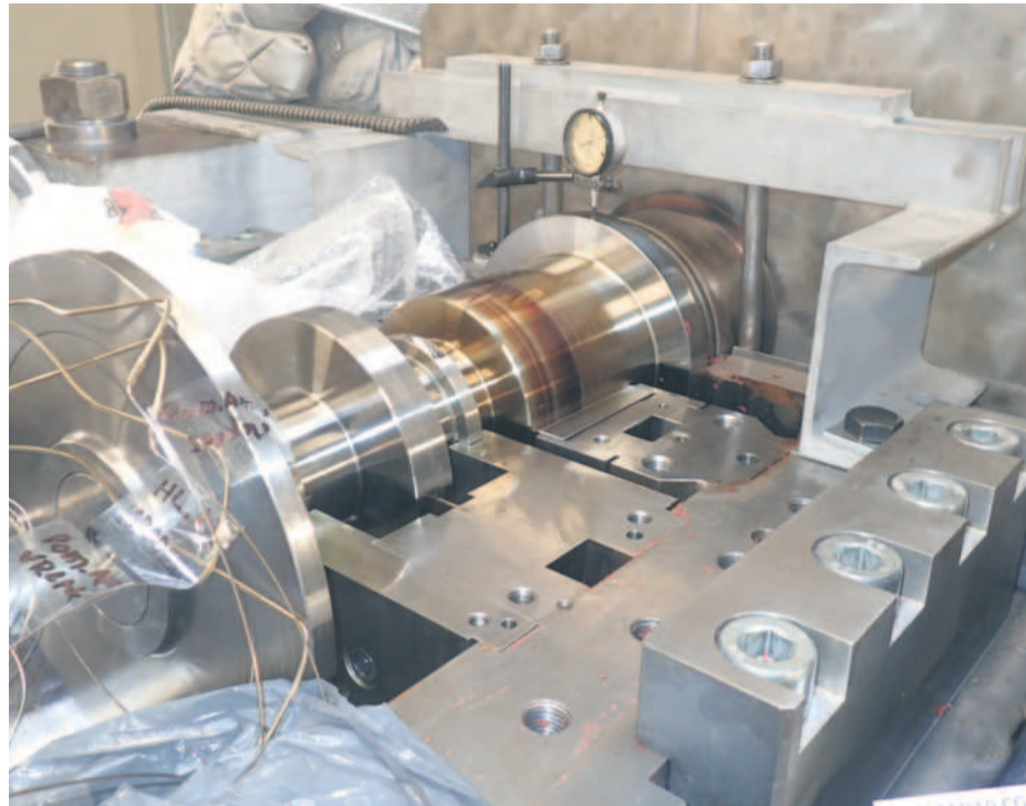
Rewizja łożysk turbiny
