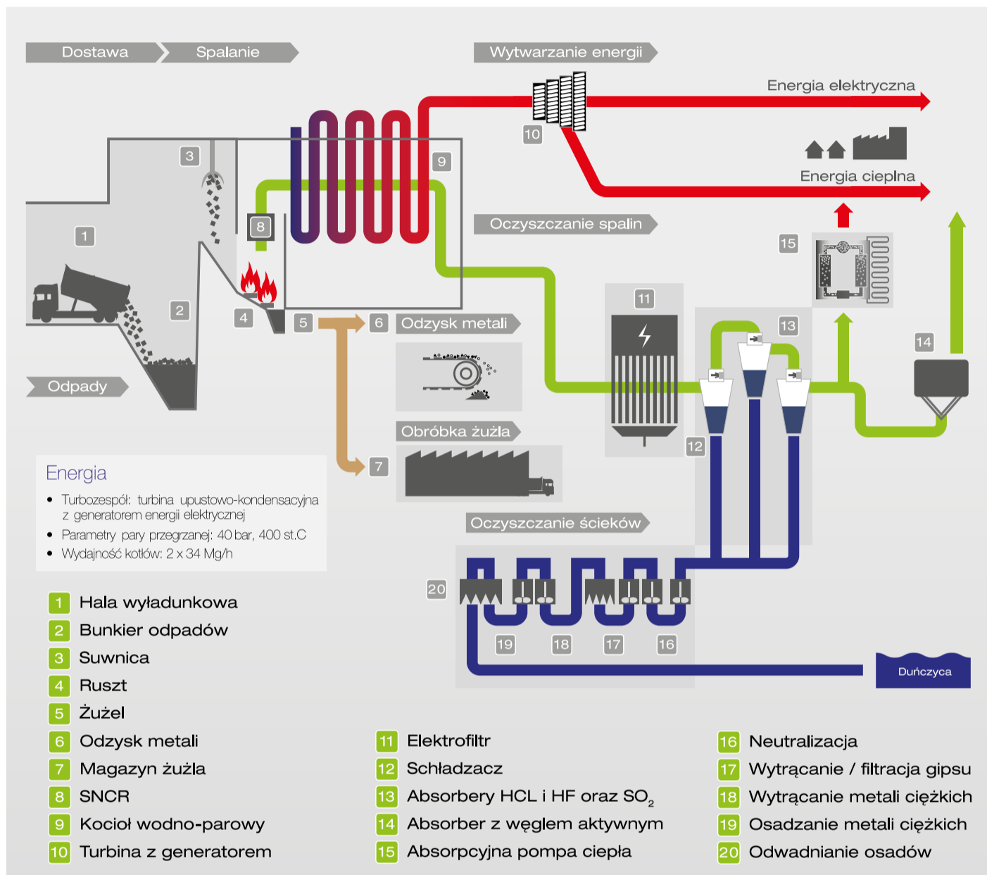
Schemat działania EcoGeneratora
