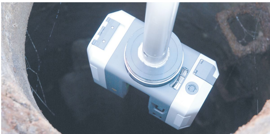
Głowica skanera wprowadzana do wnętrza studni kanalizacyjnej.
